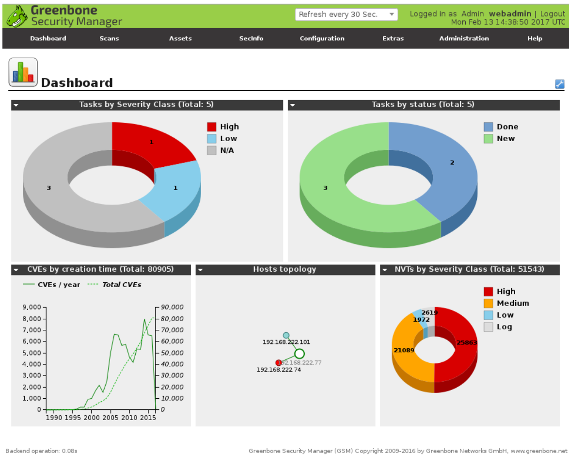
Ilustración 5. Panel principal de OpenVAS
