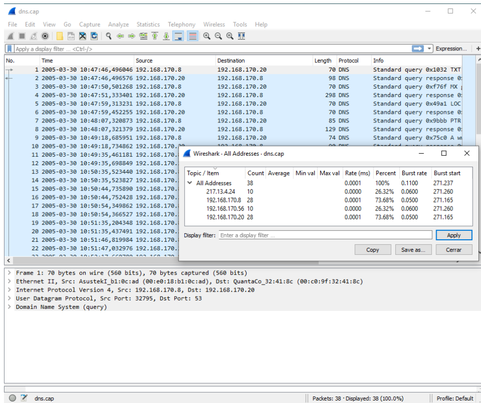
Ilustración 2. Ejemplo de activos descubiertos a través de Wireshark
