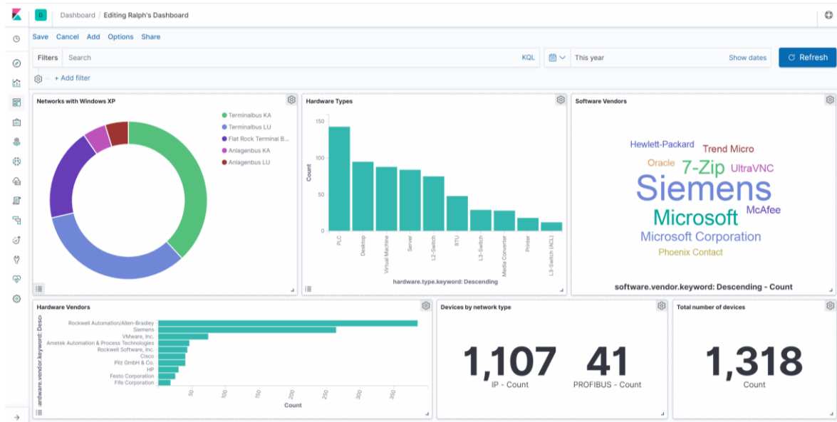
Ilustración 4. Uso de Kibana en Security Onion para un inventario de activos TO 4
